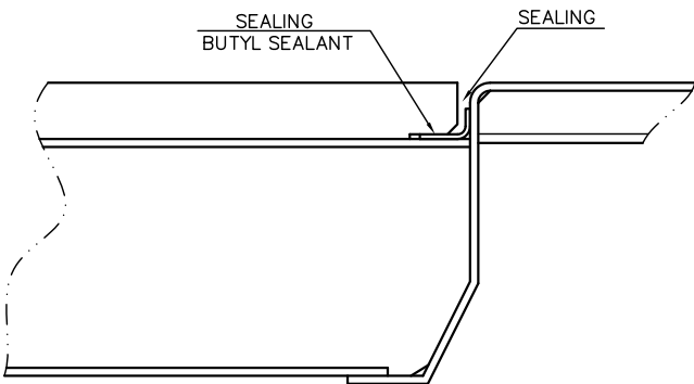
GOOSENECK 1:4
