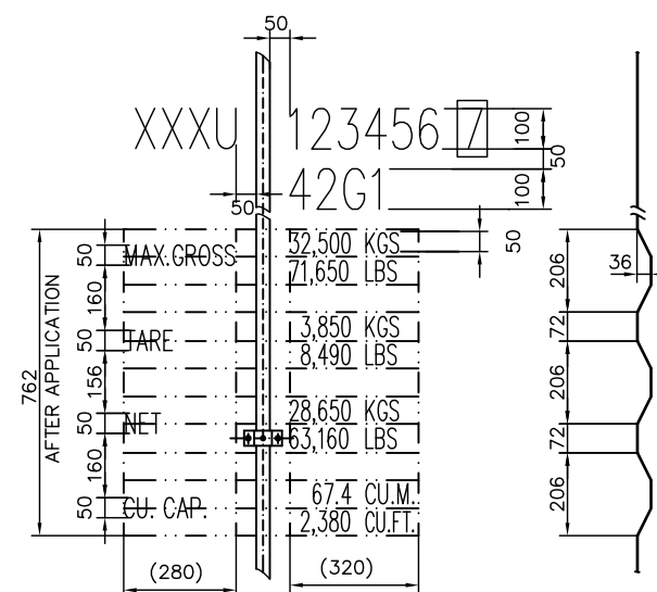
DETAIL 4;5;6 1:20
